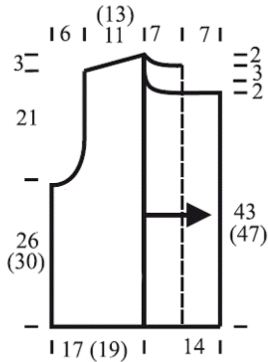
Rechtes Vorderteil und Rückenteil / Right front and back
